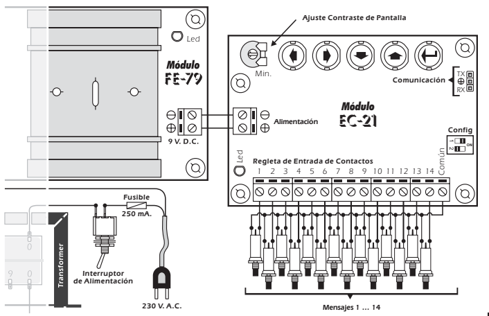
Fig. 1. Conexionado General.
