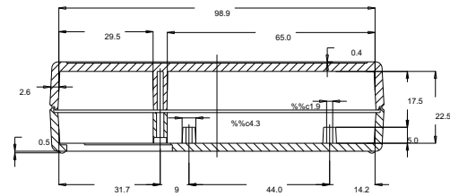
Sección A-A'
