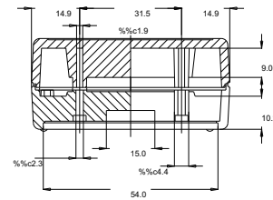
Sección B-B'
