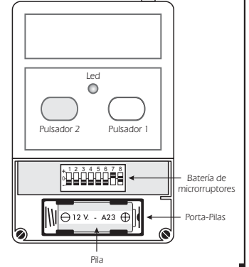
Caja abierta, sin tapa frontal.
