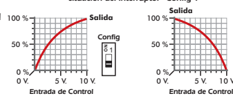
Fig. 2. Salida en función de Señal de Control y situación del interruptor "Config".
