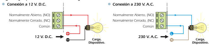
Fig. 2. Ejemplos de Conexión de la Carga.
