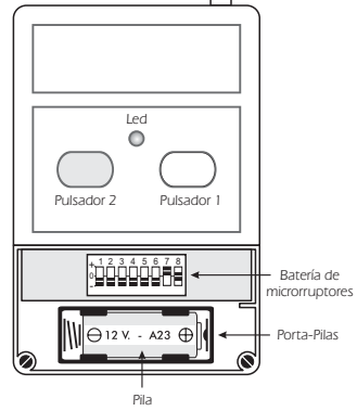
Caja abierta, sin tapa frontal.
