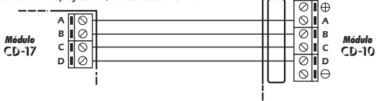
Fig. 1. Ejemplo de conexión entre la salida BCD de unidades del CD-17 y la entrada BCD de unidades de un display Cebek, en este caso el CD-10.
